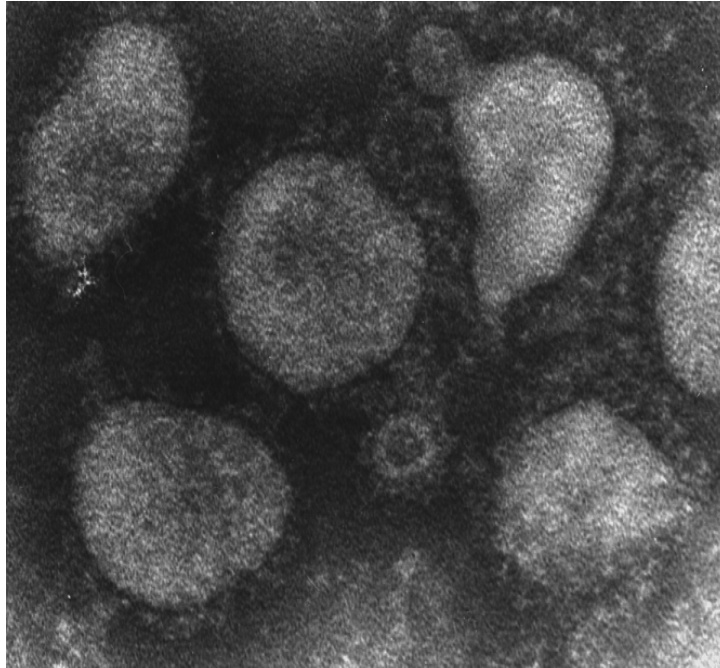
Şekil 2. Coronavirus'un elektron mikroskobu görüntüsü
