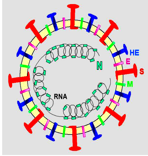
Şekil 1: Coronavirus'un şematik yapısı
